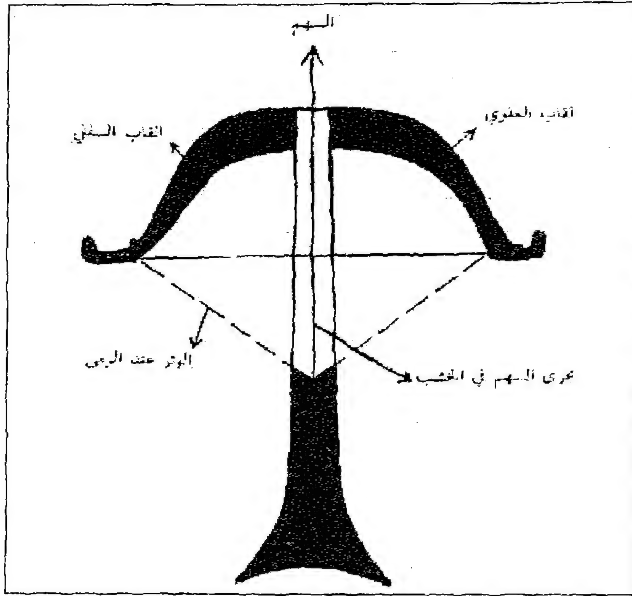
الشكل رقم (٢٤) المحتوى (قوس الأنبواب)
